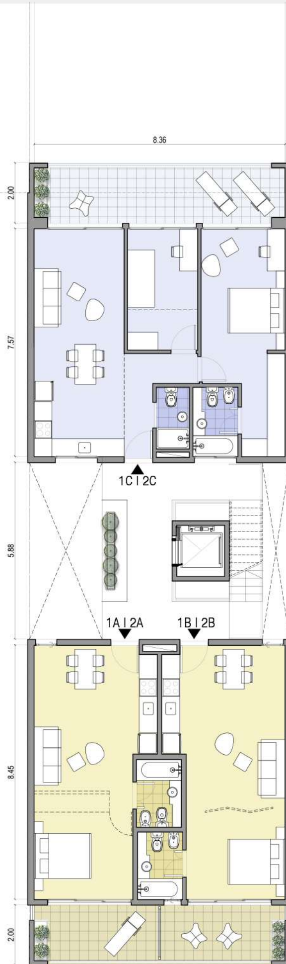
PLANTA 1° Y 2° PISO
